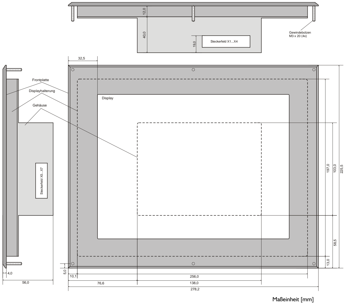
Abbildung 11: Maßzeichnung CPT800B
